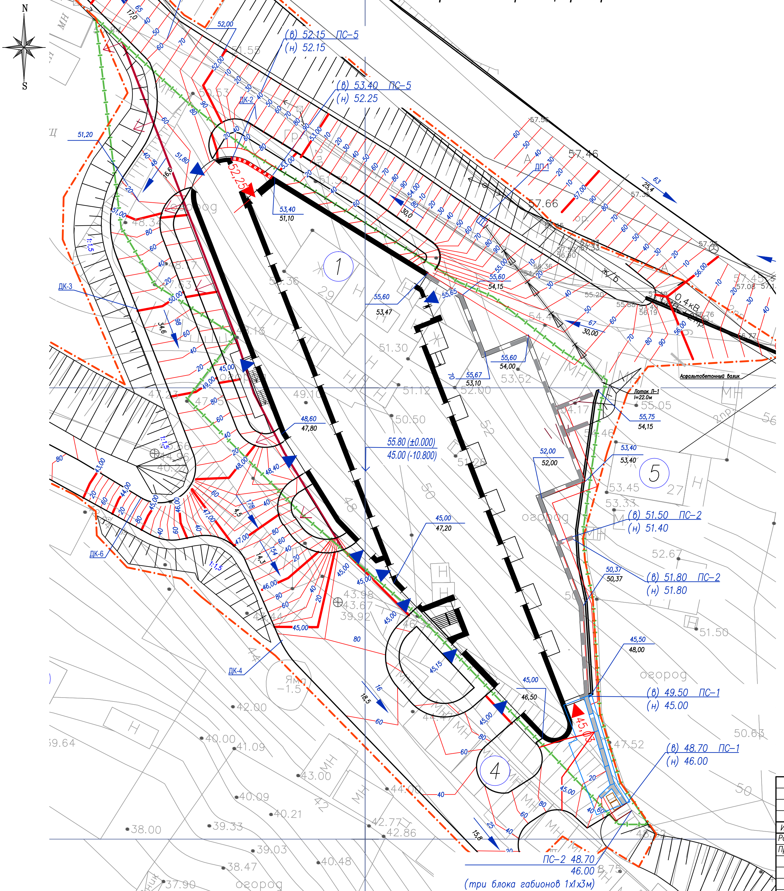
Фрагмент плана организации рельефа. М 1:250
