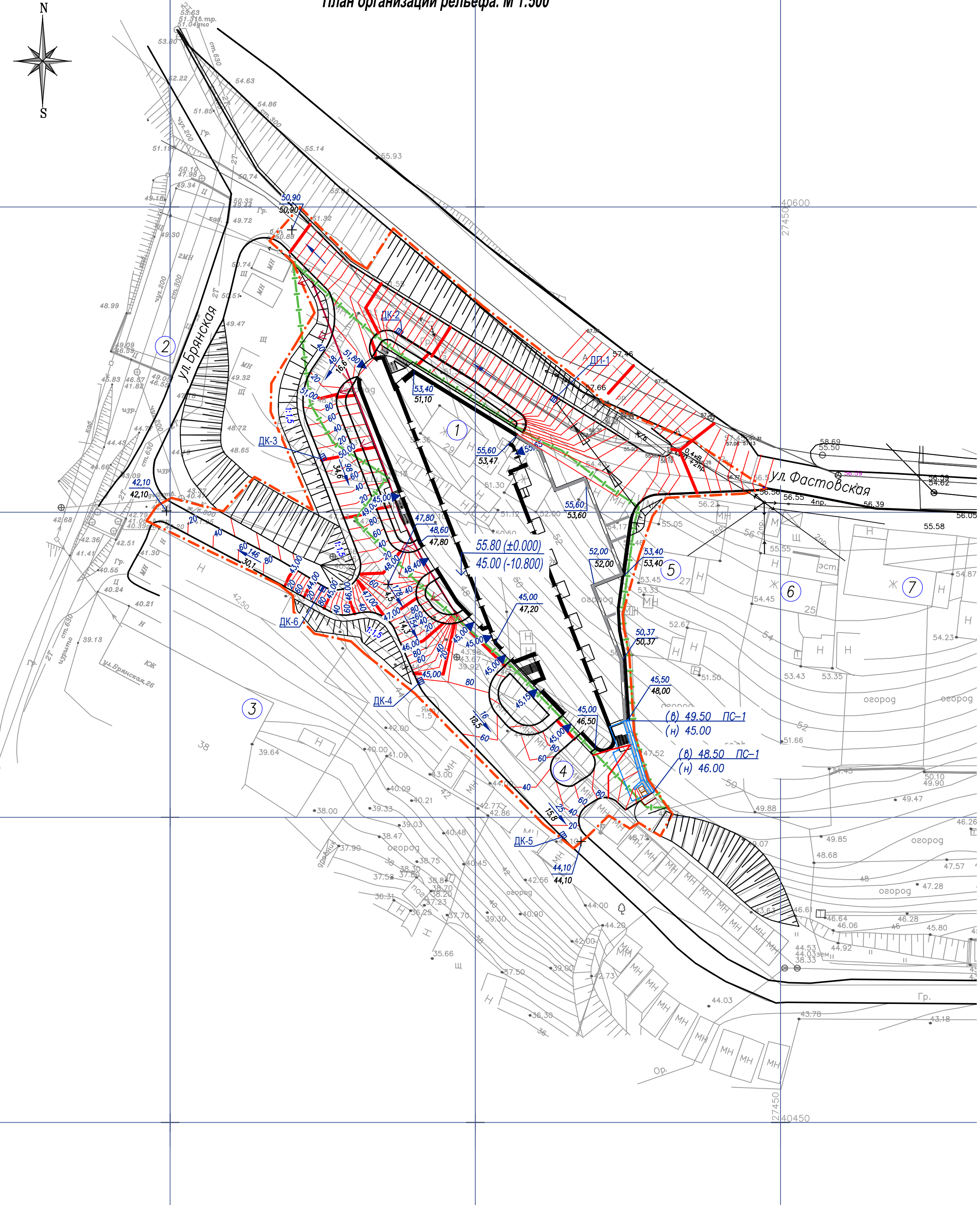
План организации рельефа. М 1:500
